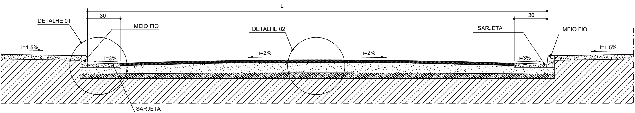
CORTE TRANSVERSAL PISTA DE ROLAMENTO - REVESTIMENTO EM CBUQ
