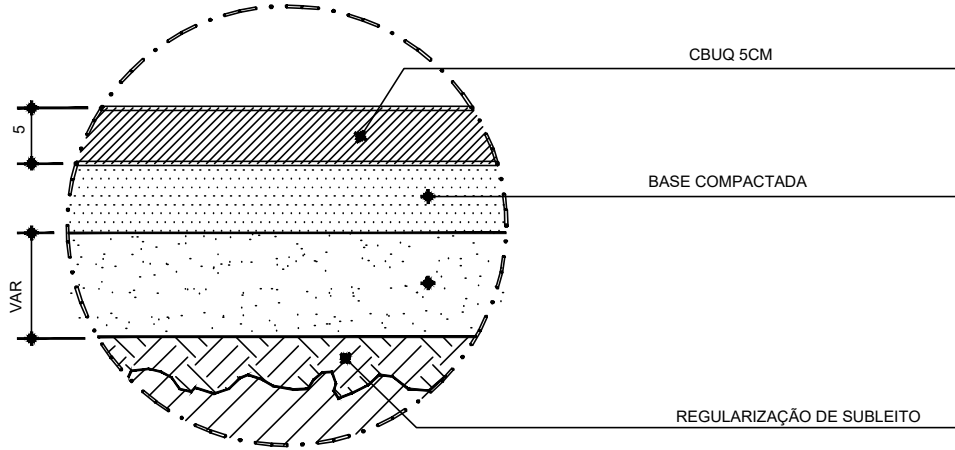
DETALHE 02 - CORTE CAMADAS - PAVIMENTAÇÃO EM CBUQ
