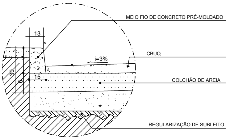
DETALHE 01 - TRECHO COM SARJETA
